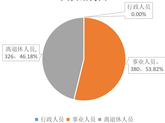
人员结构图
